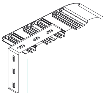
staffetta a muro per tettuccio per 21 cm, 34 cm o 47 cm wall bracket for hood for 47 cm for 21 cm, 34 cm or 47 cm Wandhalter für Schutzdach für 47 cm für 21 cm, 34 cm oder 47 cm étrier au mur pour auvent pour 47 cm pour 21 cm, 34 cm ou 47 cm soporte de pared para tejado para 47 cm para 21 cm, 34 cm o 47 cm soporte de parede para telhado para 47 cm para 21 cm, 34 cm ou 47 cm
