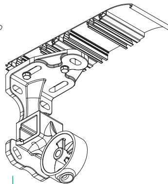
staffa renoir con disco renoir bracket with disk Renoir Konsole mit Scheibe support renoir avec disque soporte renoir com disco suporte renoir com disco
