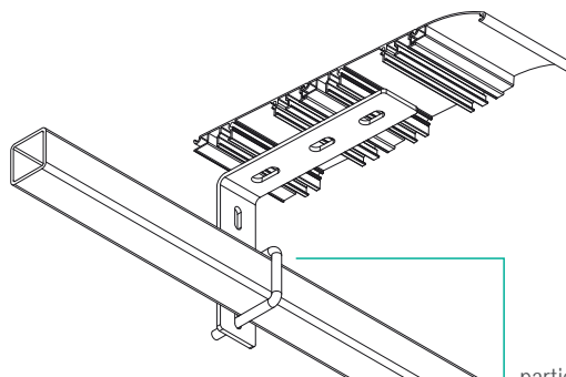
staffa renoir con disco renoir bracket with disk Renoir Konsole mit Scheibe support renoir avec disque soporte renoir com disco suporte renoir com disco
