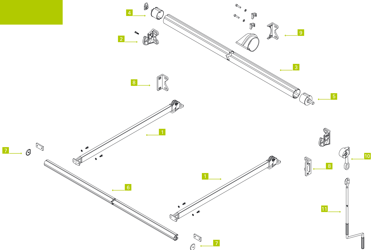
braccio Vanvitelli - Vanvitelli arm - Gelenkarm Vanvitelli - bras Vanvitelli
