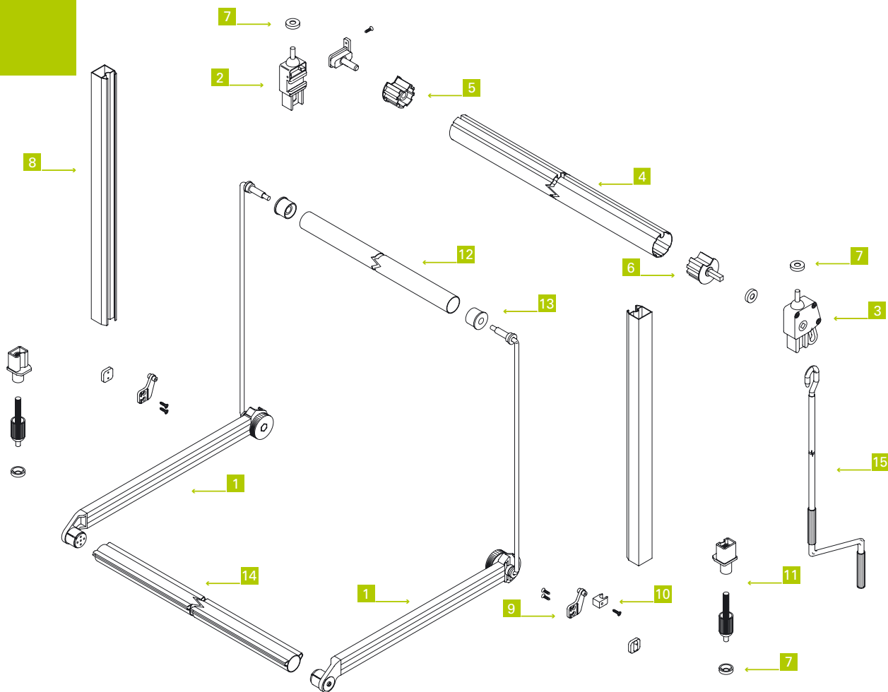
braccio Canaletto - Canaletto arm - Gelenkarm Canaletto - bras Canaletto
