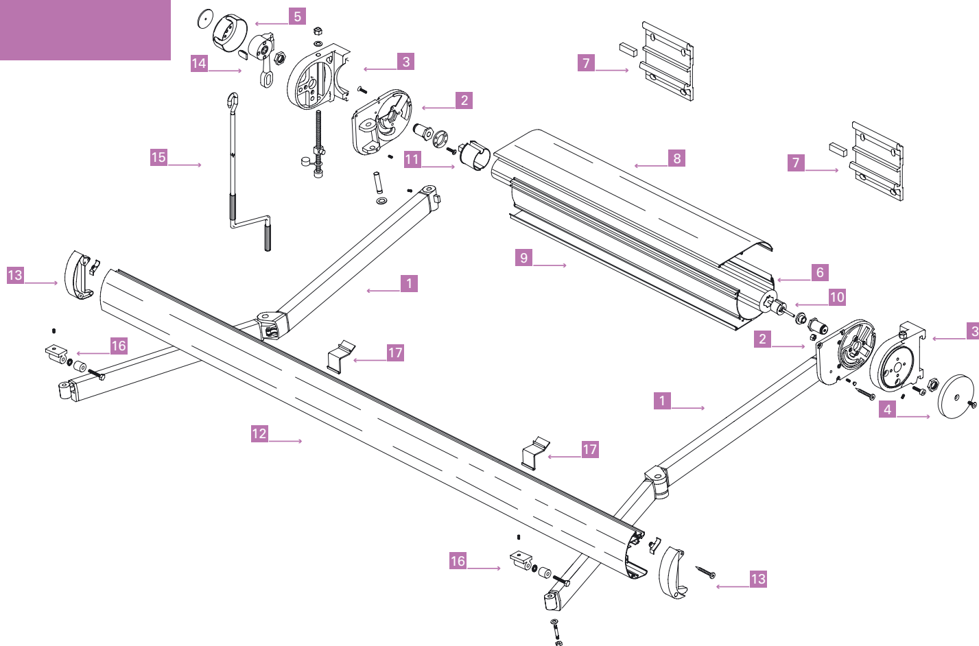
braccio Lybra - Lybra arm - Gelenkarm Lybra - bras Lybra
